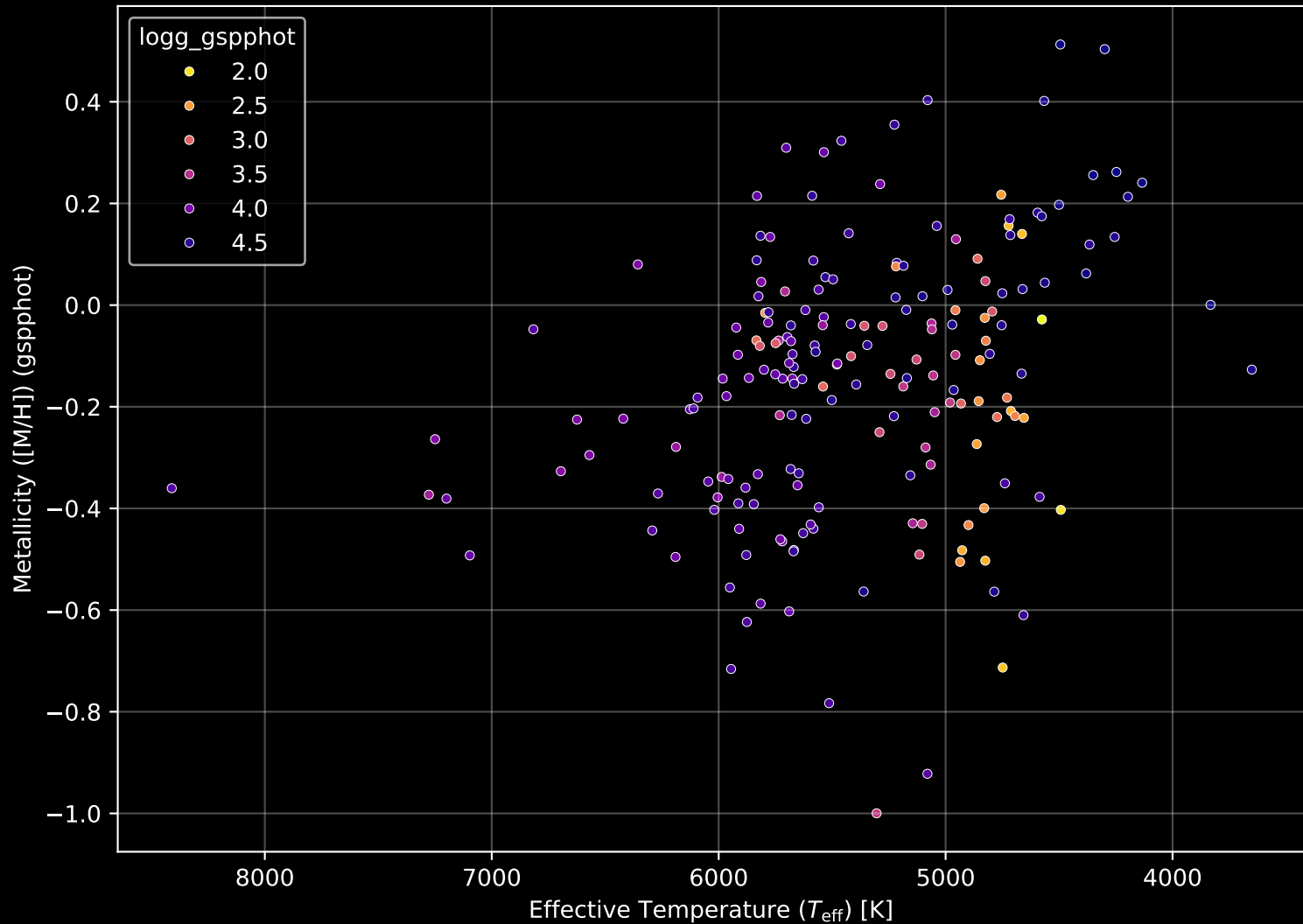
APOGEE DR17 Field: [267-34-O_TESS] Stellar Population Parameters (n= 192)
